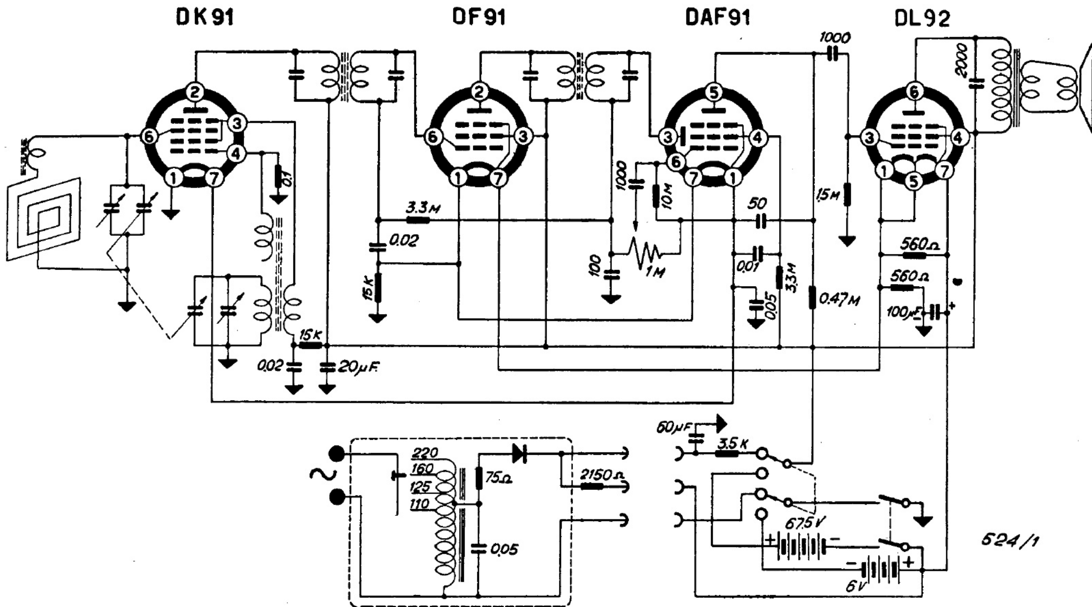
MINERVA RADIO - Mod. 524/1. Supereterodina tascabile a 4 valvole. Onde medie da 190 a 570 m. Alimentazione con batterie di pile a secco incorporate e con corrente alternata da 110 a 220 V. Alimentatore con rettificatore a selenio, separato. Media frequenza 468 kc. Consumo 13 W in alternata. Larghezza cm 25, altezza cm 8,5, profondità cm 12. Peso kg 1,600.
